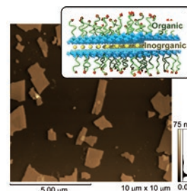
図 1 ポリマー修飾無機ナノシートの顕微鏡像
