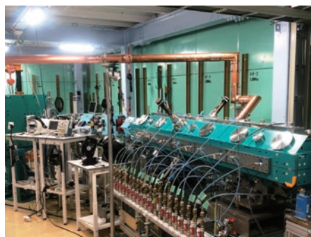
図2 理研小型中性子源システム2号機（理化学研究所との共同開発）
