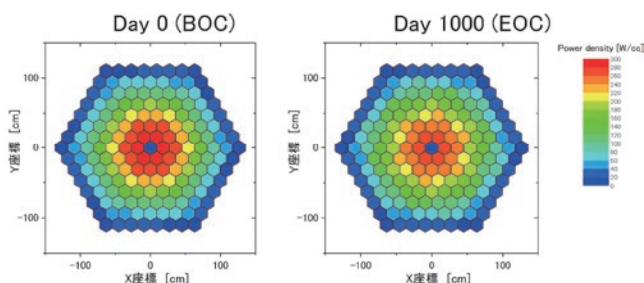
図 1 回転型燃料シャッフルブリードバーン型高速炉の炉内出力分布
