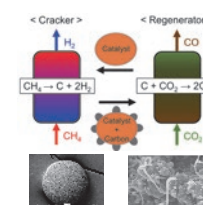
図 3 炭素循環利用化学ルーピング Fig. 3 Chemical looping for circular use of carbon dioxide
