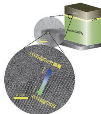
図 1 Cu(In,Ga)Se 2 太陽電池
