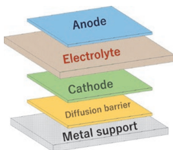
図 1 金属支持 SOC 構造
