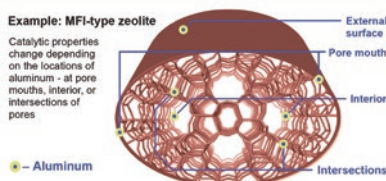
図 1 ゼオライト骨格内 Al 原子の位置
