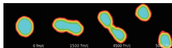
図 2 微視的核反応モデルを用いた ^{236}\text{U} 核分裂の模擬計算
