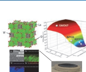
図 1 高効率プロトン伝導型燃料電池 Fig. 1 Highly efficient proton-conducting fuel cell
