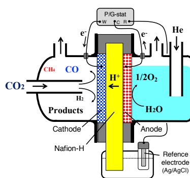
図 1 CO 2 気相電解
