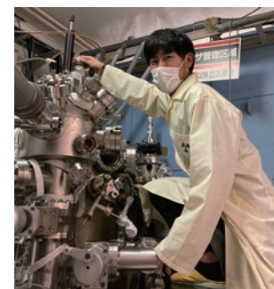
図 1 高エネルギー加速器研究機構フォトンファクトリー BL27A の XPS チャンバー
