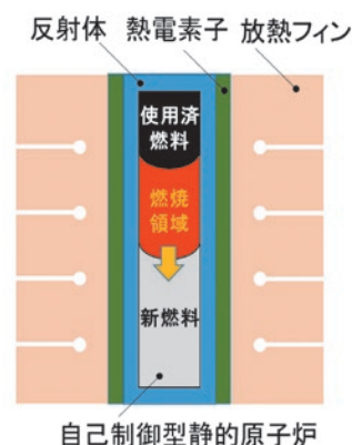
図 1 宇宙探査用小型原子炉システムの概念図
