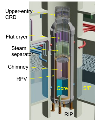
図 1 LLBWR の原子炉概念 Fig. 1 Reactor Concept of LLBWR
