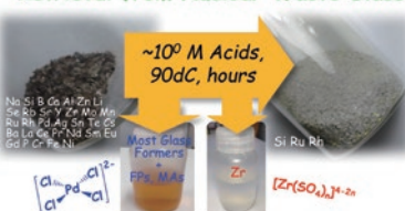
図 3 将来的核変換のための放射性廃棄物ガラス固化体湿式処理技術開発。
