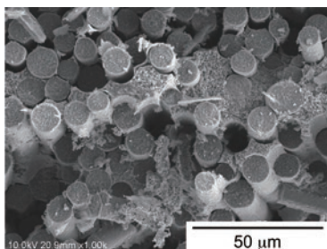
図1 炭化ケイ素繊維強化炭化ケイ素基 (SiC/SiC) 複合材料の微構造 SEM 写真
