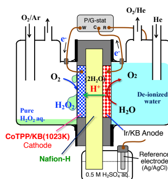
図 2 水と空気からの過酸化水素合成
