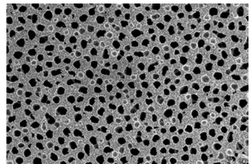
図 3 複合金属水素分離膜の SEM 像
