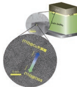
図 1 Cu(In,Ga)Se 2 太陽電池 Fig. 1 Cu(In,Ga)Se 2 solar cells
