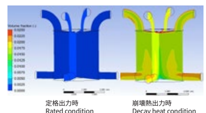
図 2 炉心内ボイド率分布変化
