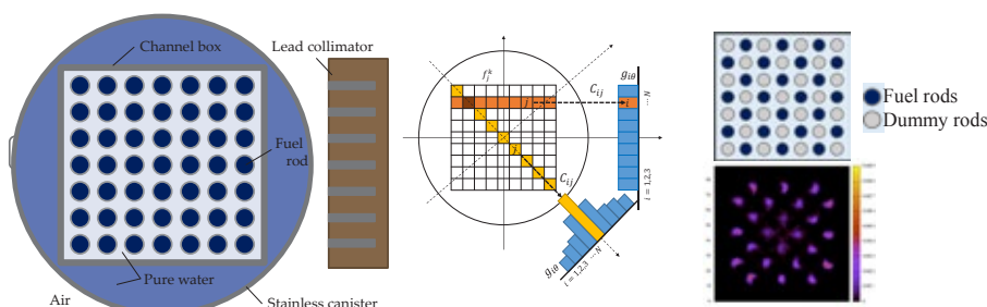
図2 パッシブγ断層撮影法を用いた非破壊測定技術の燃料欠損検知への応用
