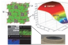
図 1 高効率プロトン伝導型燃料電池 Fig. 1 Highly efficient proton-conducting fuel cell
