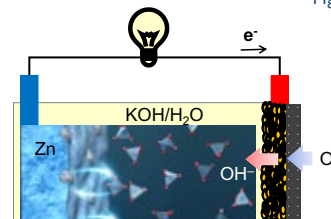
図 2 亜鉛空気電池
