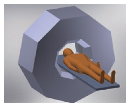
図 2 BNCT 用線量評価システムの概念図
