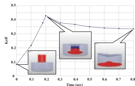
図 2 水中にデブリが落下したときの実効増倍率の変化
