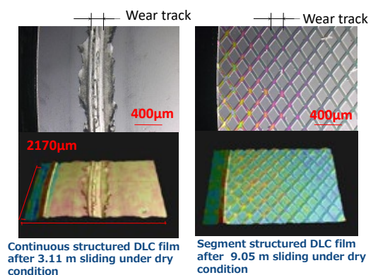
図 1 微細表面構造（セグメント構造）DLC 膜の提案
