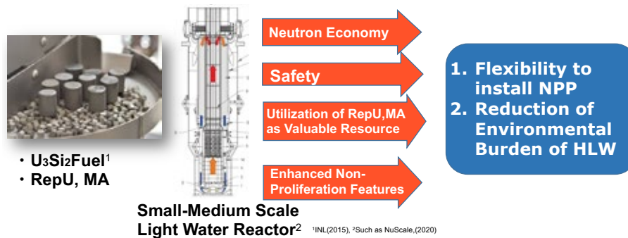
図1 ケイ化物燃料を用いた高安全・核不拡散性を有する中小型軽水炉概念
