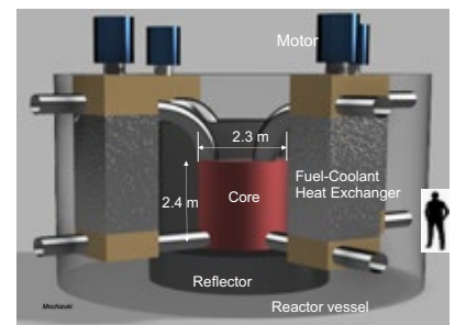
図 1 溶融塩高速炉 MCSFMR の炉心概要
