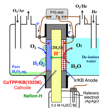
図 2 水と空気からの過酸化水素合成 Fig. 2 Hydrogen peroxide production from water and air
