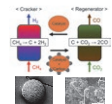
図 3 炭素循環利用化学ループ Fig. 3 Chemical looping for circular use of carbon dioxide
