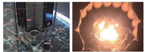
図3 原子炉芯構造物とコールドクルーシブルによる燃料系デブリ模擬溶融試験
