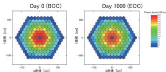
図 1 回転型燃料シャッフルブリードバーン型高速炉の炉内出力分布
