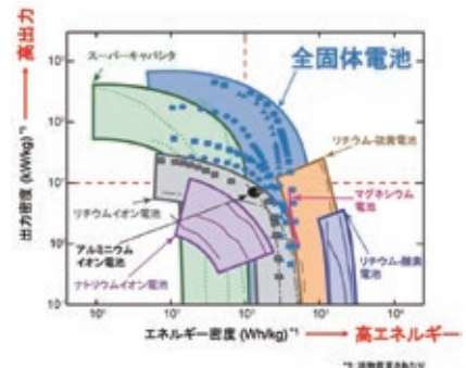
図2 固体電解質を用いた全固体電池の優れた出力特性
