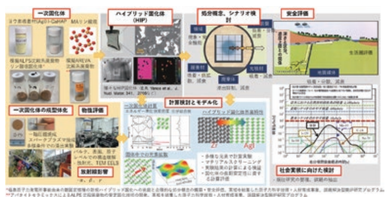
図 2 福島第一原子力発電所事故由来の難固定核種の新規ハイブリッド固化
